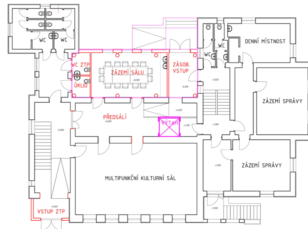
přízemí po přestavbě
